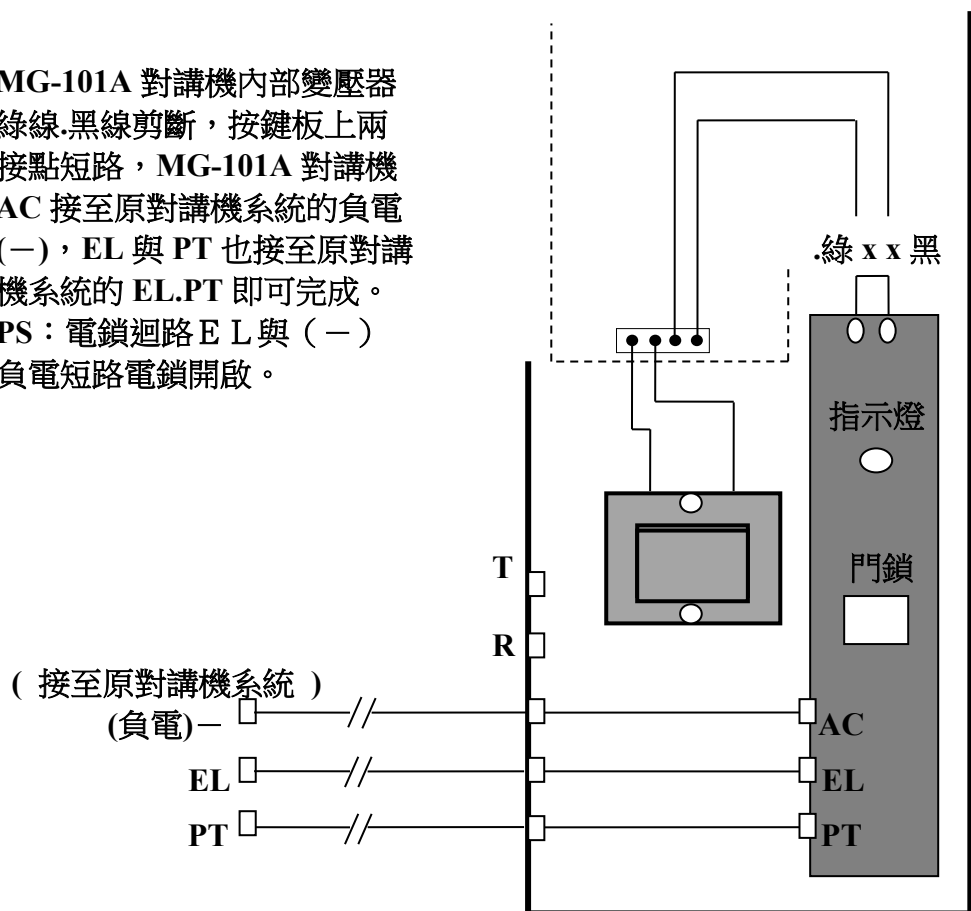
MG-101A 對講機內部
